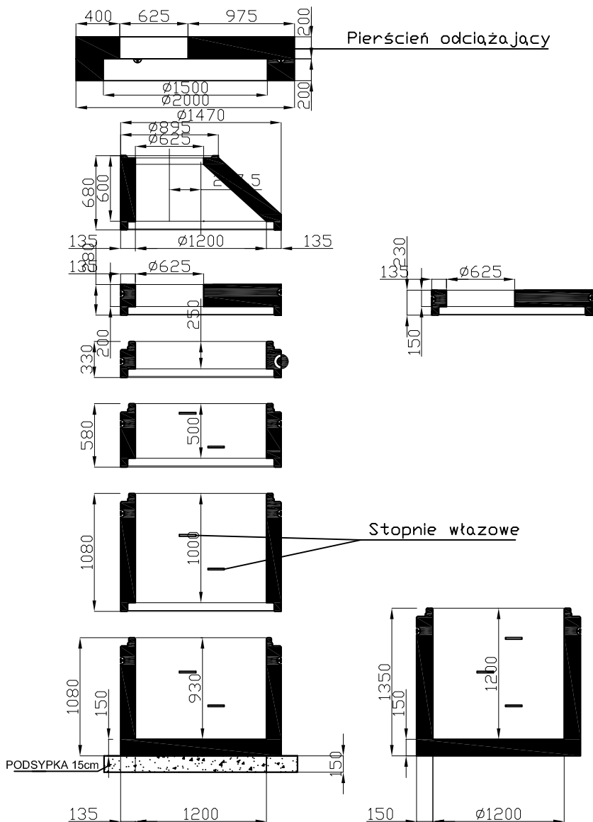
Studnia kanalizacyjna \varnothing 1200
