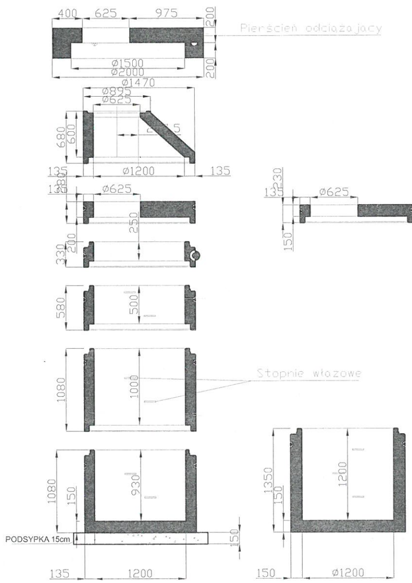
Studnia kanalizacyjna \varnothing 1200
